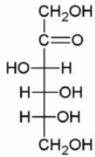
Fructose
